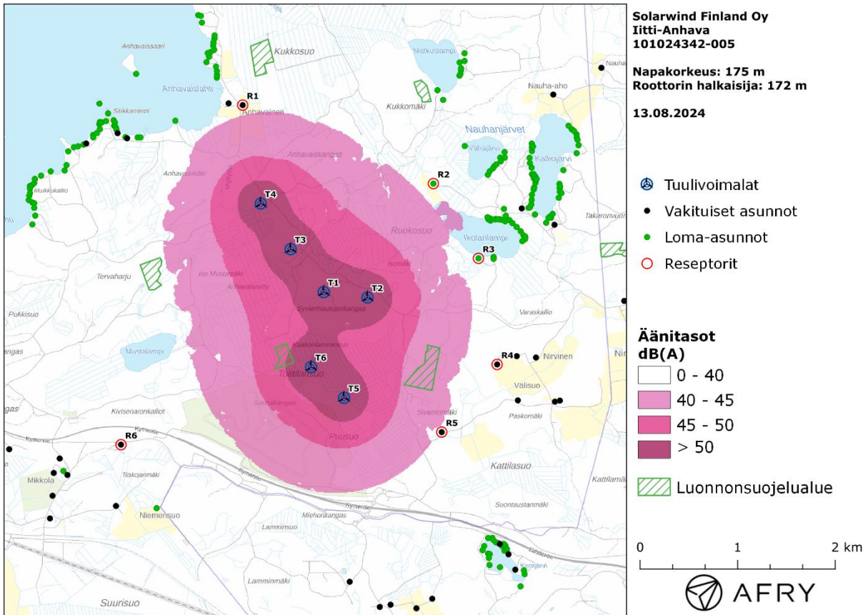
Kuva 4: Keskiäänitasot LAeq Anhavan tuulivoimapaiston hankealueella.
